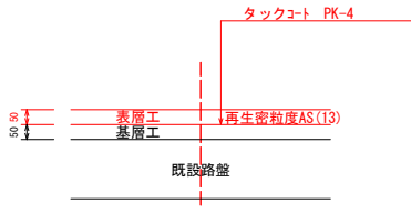
施工要領図
